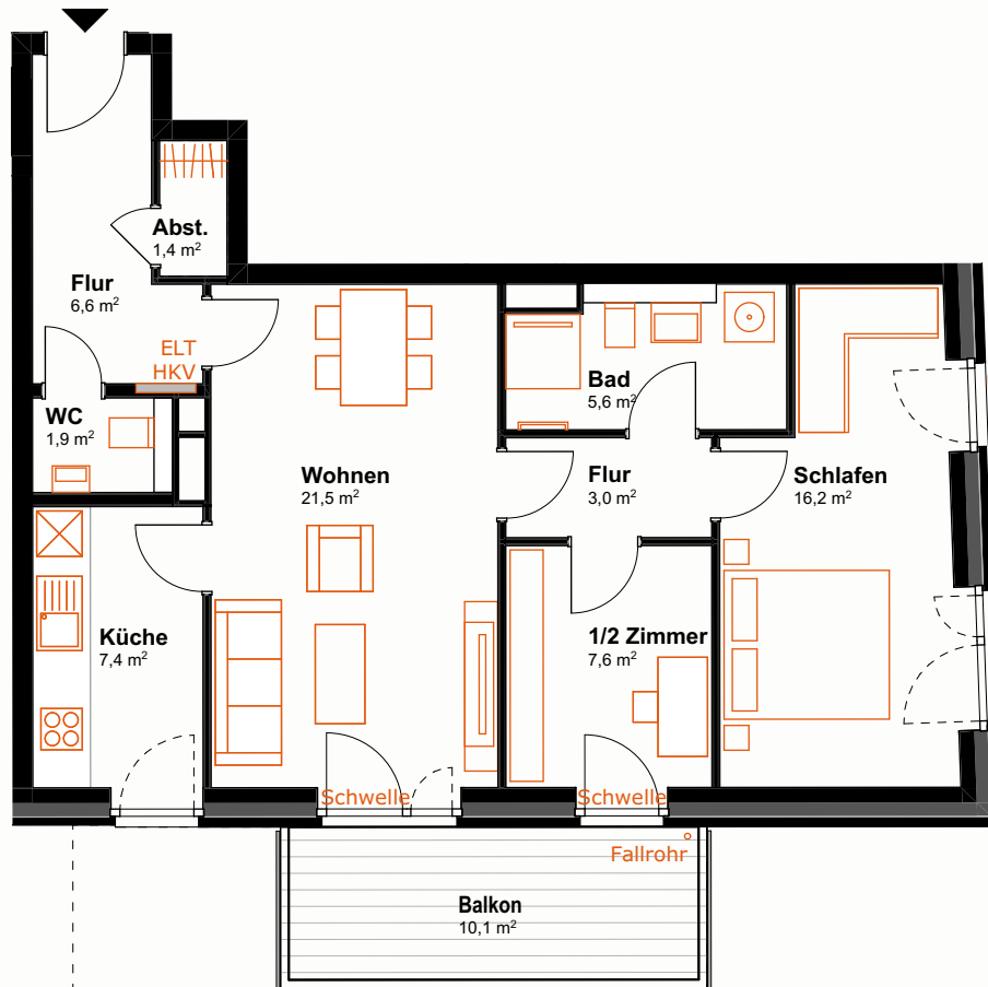
Geschossplan
