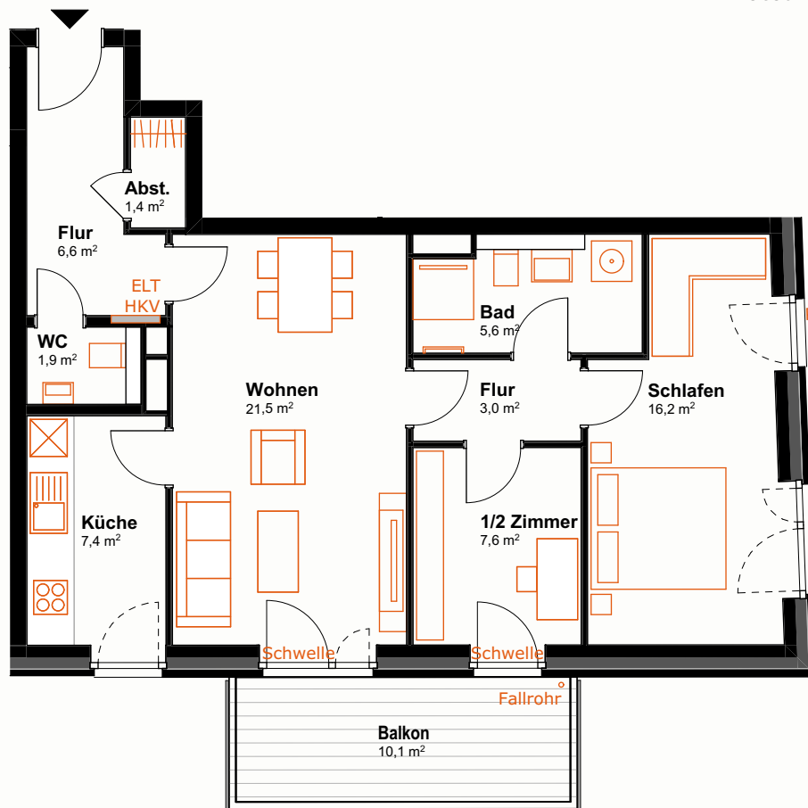
Geschossplan
