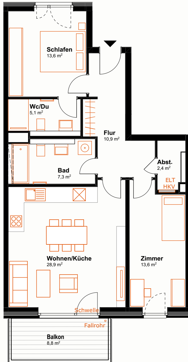
Geschossplan
