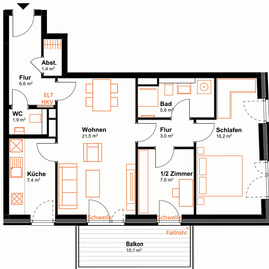
Geschossplan
