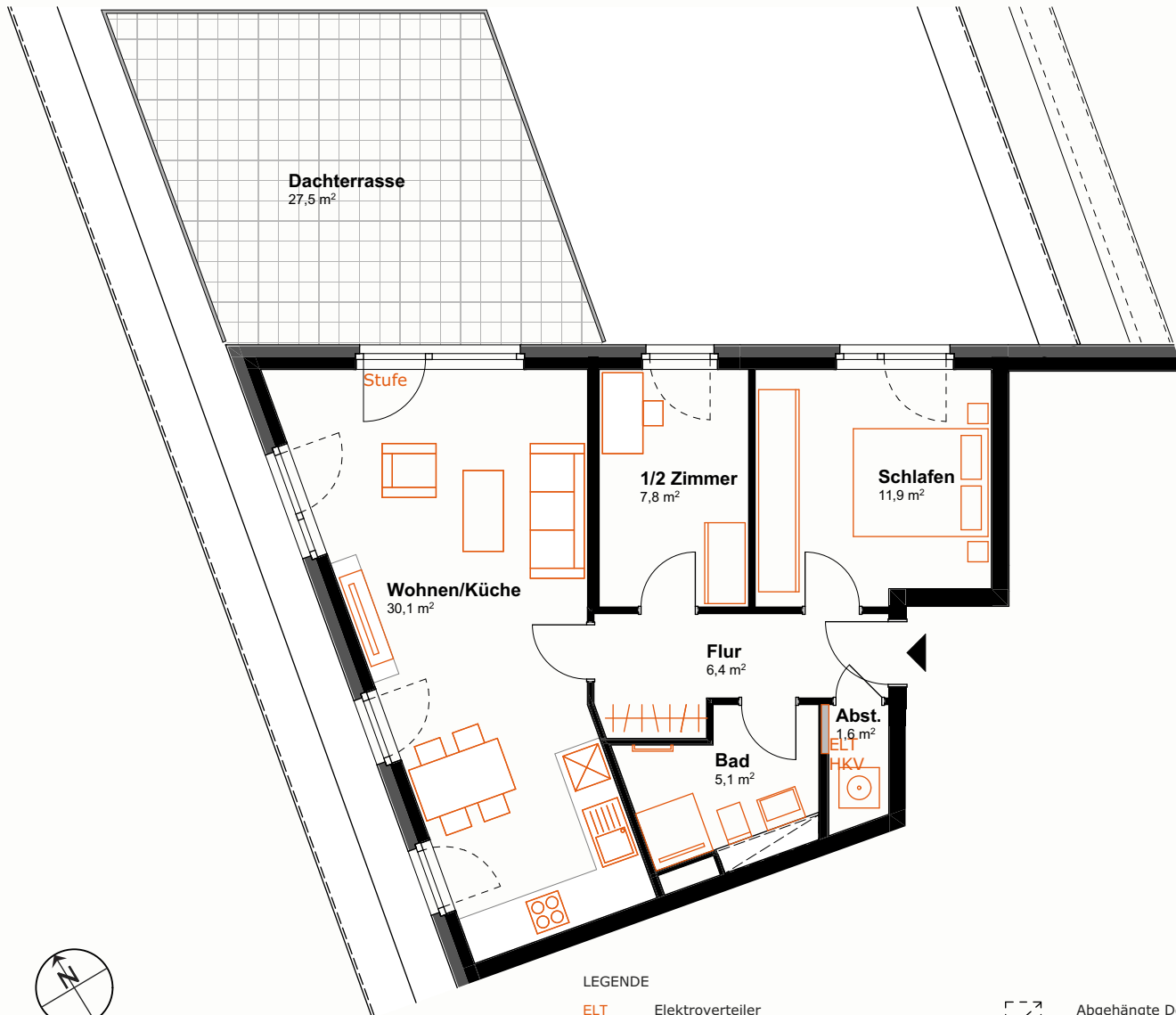
Geschossplan
