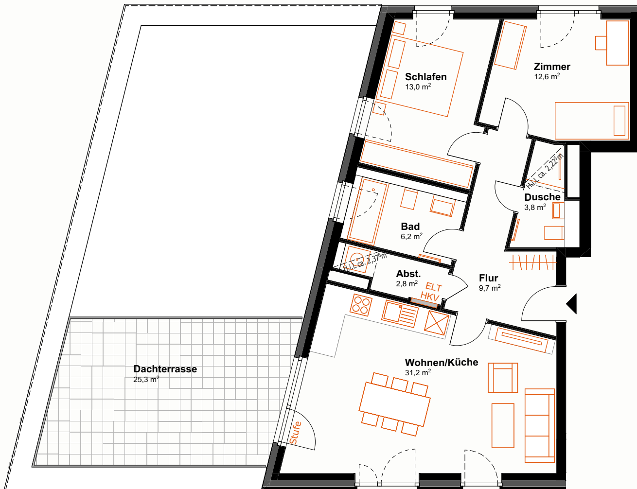
Geschossplan
