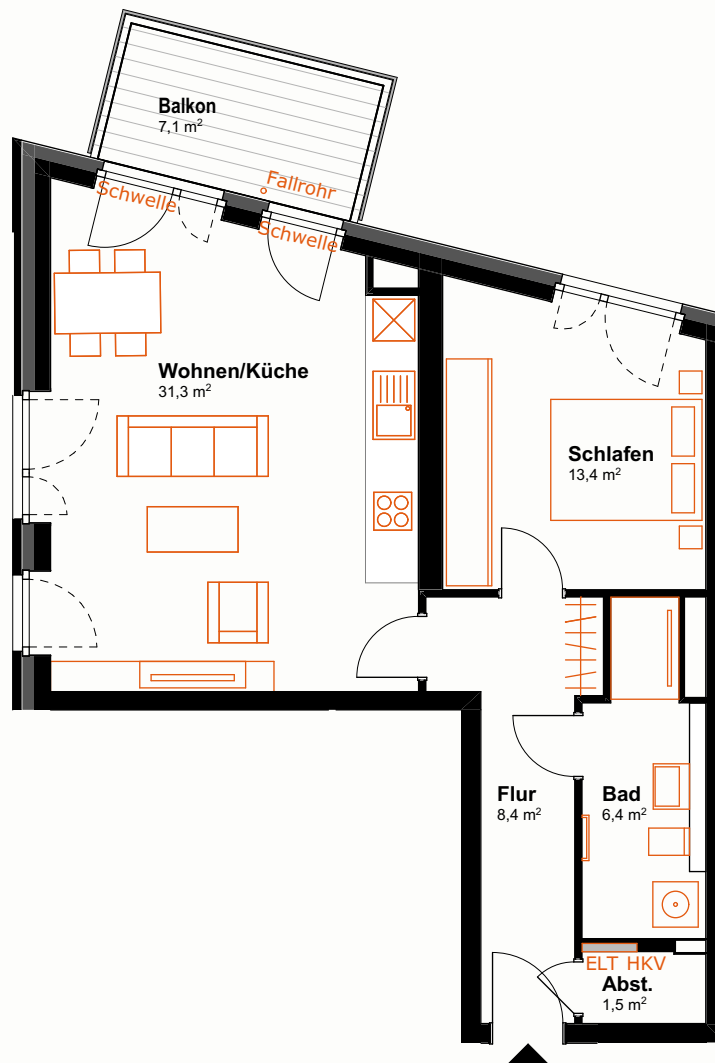
Geschossplan
